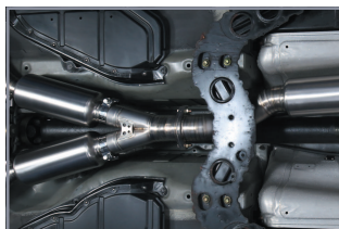
最低地上高に配慮したレイアウト
