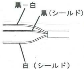
車両配線
