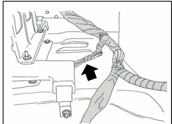
図1 ハーネス切断位置
