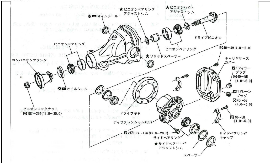
リヤ分解図
