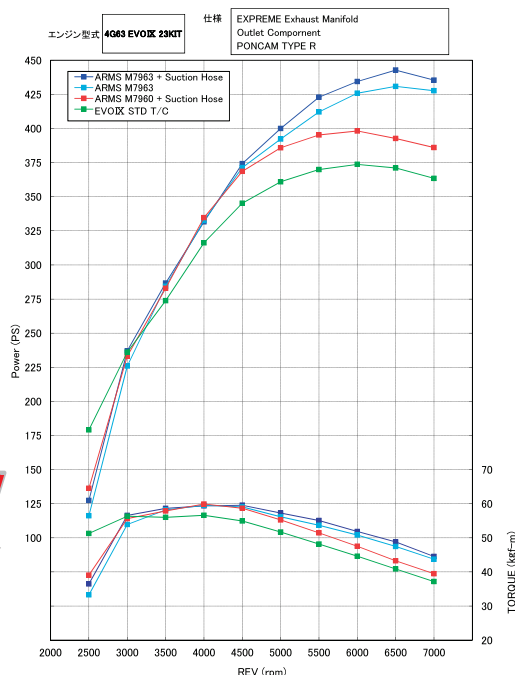
エンジン試験表
