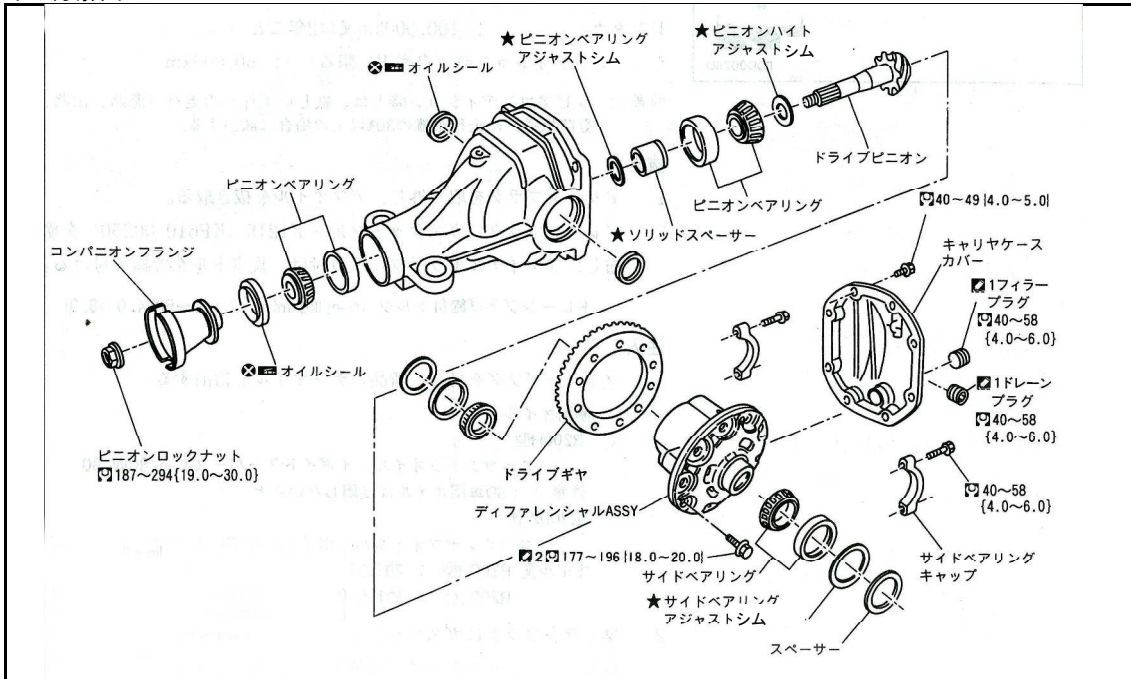
リヤ分解図
