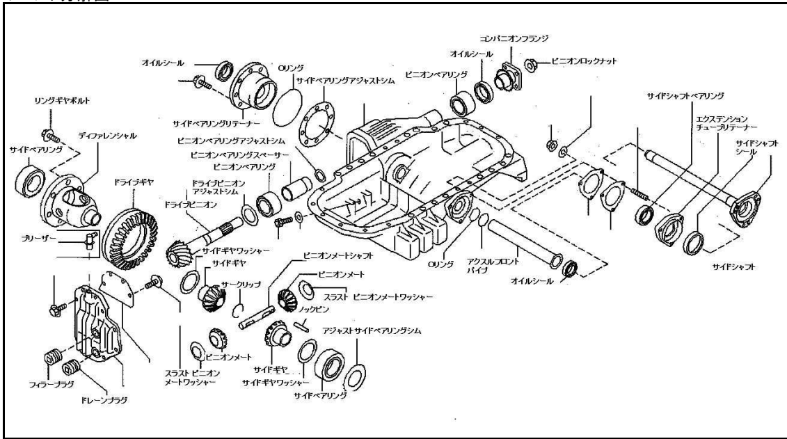
フロント分解図
